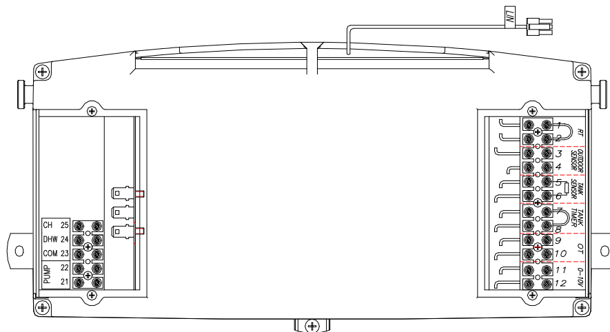
Схема 3.9.1 Електрическо контролно табло
