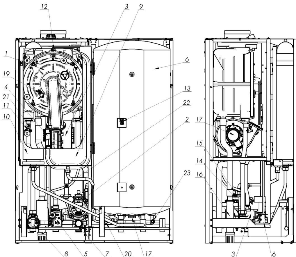
Схема 2.2.1.1. Основни части на INTEGRA COMFORT
