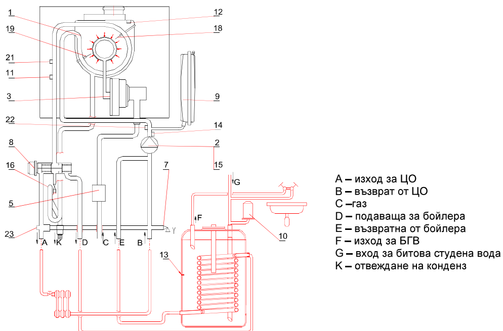
Схема 2.2.1.2. Схема за работата на котела
