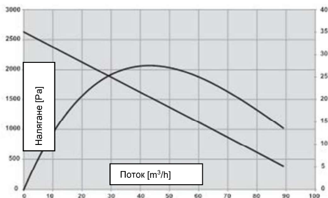
Схема 4.3.1. Характеристики на вентилатор тип PX 118
