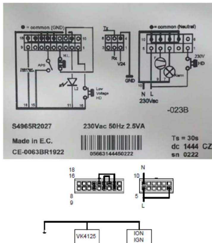
Схема 8. Ел. подключение на уреда при електроника S 4965R2027
