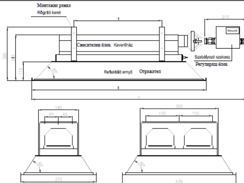
Схема 1. Основни характеристики на газови инфрачервени излъчватели
