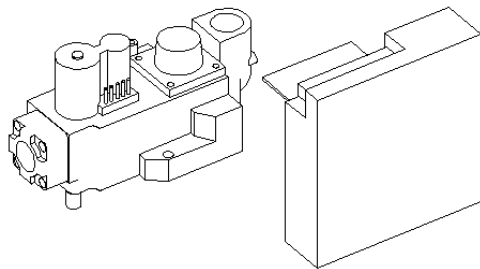
Схема 5. Сглобяване на газовия клапан и електрониката
