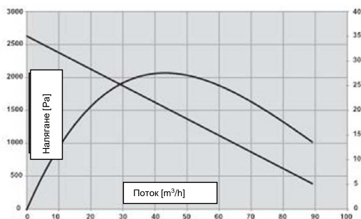
Схема 4.4.1. Характеристики на вентилатор тип PX 118
