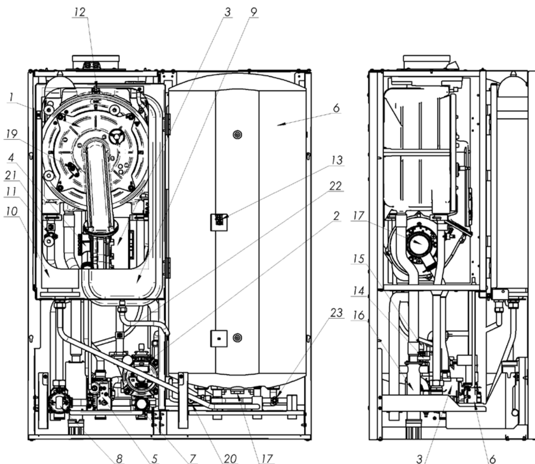
Схема 2.2.1.1. Основни части на ECOCONDENS INTEGRA II PLUS
