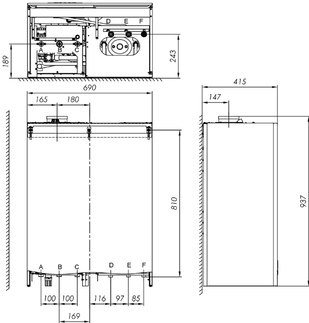
Схема 3.3.1 Монтажни размери на котела
