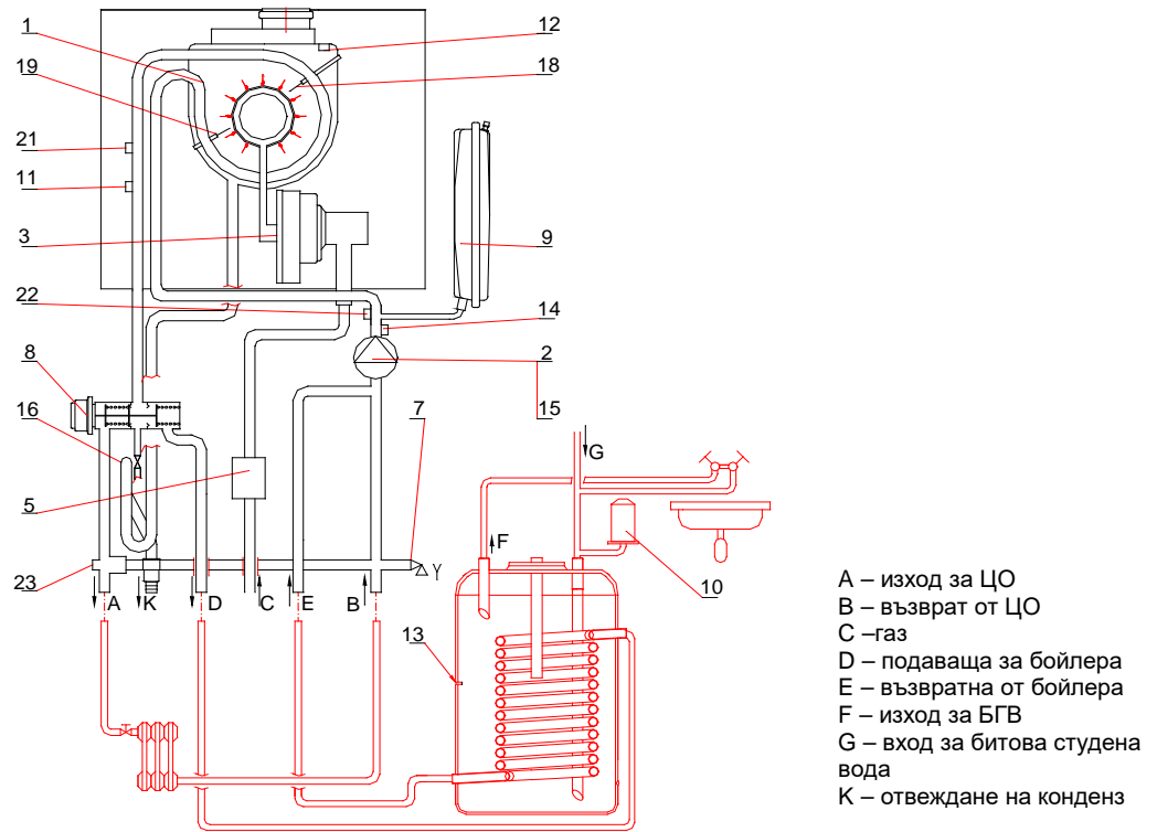
Схема 2.2.1.2. Схема за работата на котела
