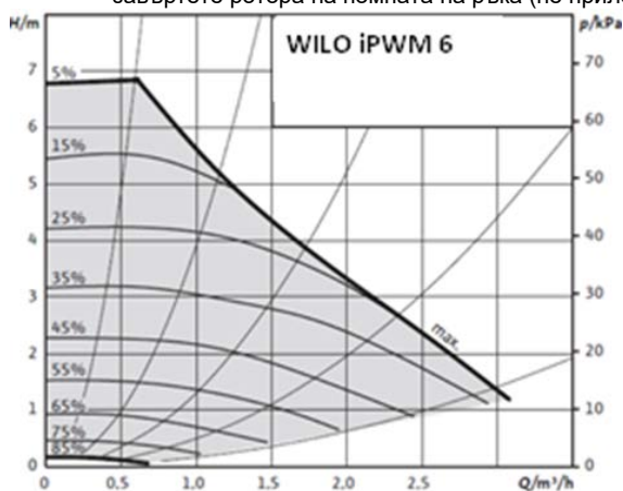
Схема 6.1.5.1 Характеристика на помпата
