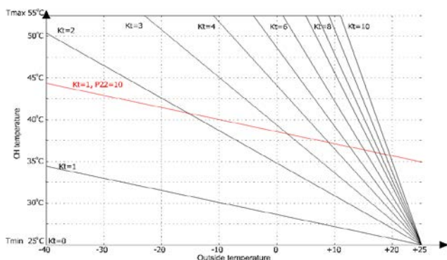
Схема2.4.2.1 Крива на затопляне (стандартна инсталация)
